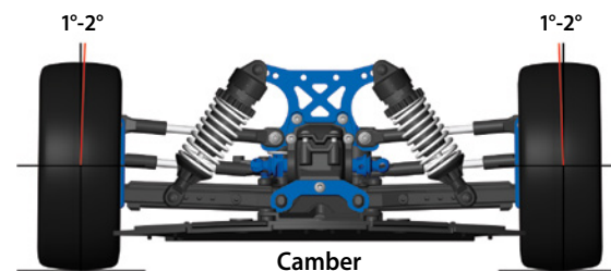
Camber
